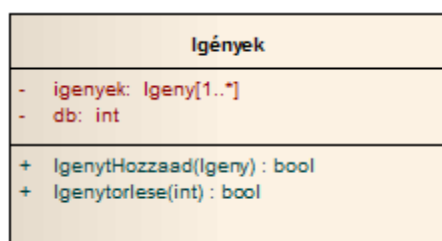
59. ábra: Metódusok jelölése osztálydiagramon
