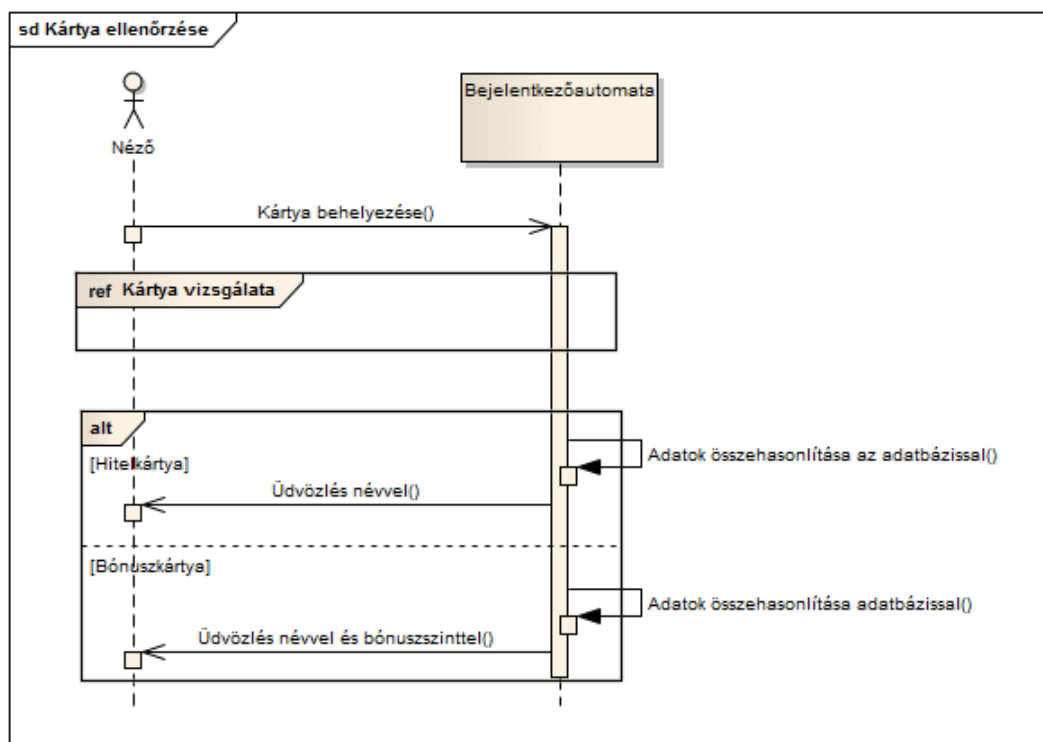
81. ábra: Kártya ellenőrzése szekvenciadiagram operátorokkal
