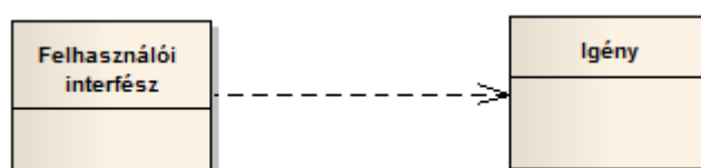
60. ábra: Függőség jelölése
