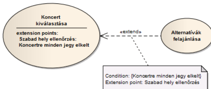
19. ábra: Kiterjesztési pont a Koncert kiválasztása folyamatban
