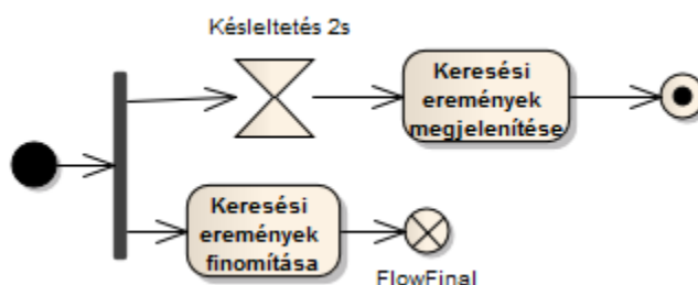
43. ábra: A folyamat záró csomópont csak az adott folyamat futására van hatással
